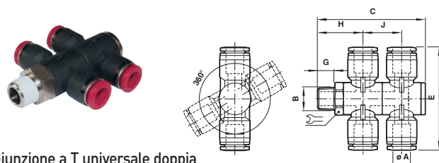
Giunzione a T universale doppia
