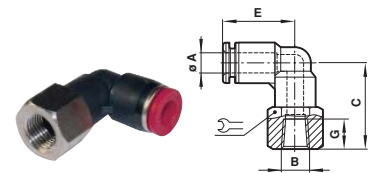
Gomito girevole 90° (filetto femmina)
