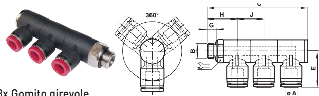
3x Gomito girevole
