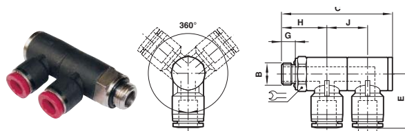
2x Gomito girevole
