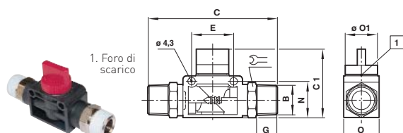
3/2 Valvola di esclusione
