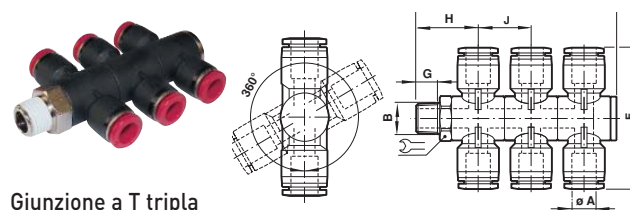
Giunzione a T tripla
