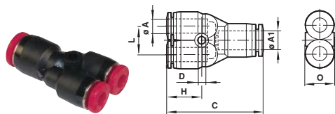
Giunzione a Y
