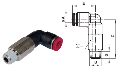
Gomito girevole 90° [Esteso]
