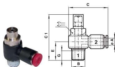
Banjo protetto (Regolazione in uscita)
