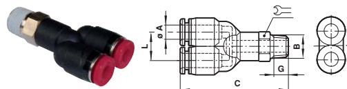
Giunzione a Y girevole
