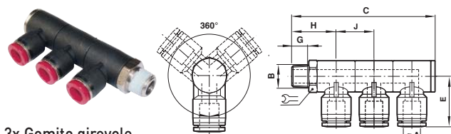
3x Gomito girevole
