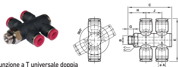
Giunzione a T universale doppia
