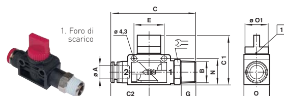
3/2 Valvola di esclusione
