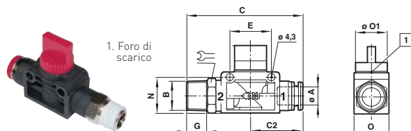
3/2 Valvola di esclusione
