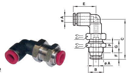
Gomito giunzione passaparete
