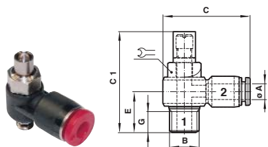
Regolatore di flusso Banjo protetto (Regolazione in uscita)
