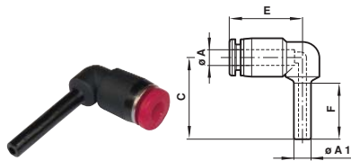
Giunzione a gomito a codolo
