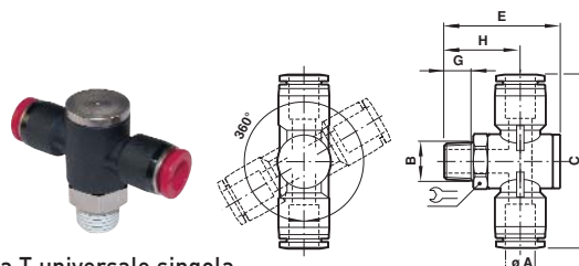
Giunzione a T universale singola
